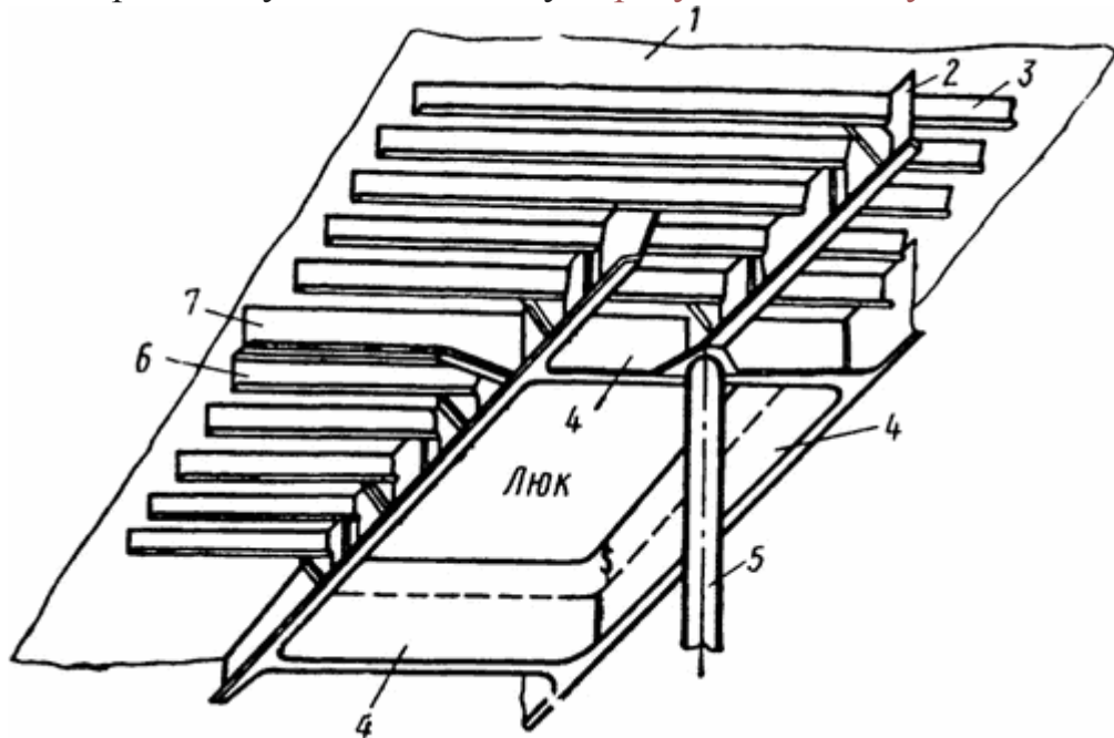
Конструкція палуби (вид з трюму) суховантажного судна (поперечна система набору): 1 - настил палуби, 2 - карлингсами, 3 - бімс, 4 - поздовжній і поперечний комінгси люка, 5 - пілерсів, 6 - полубімс, 7 - кінцевий бімс
